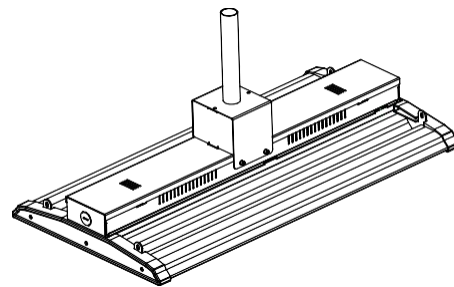
pendant mount
