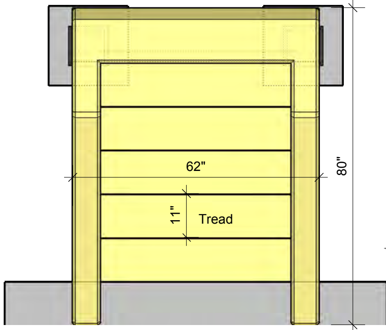
2 Top View A00 Scale: 1/2"=1'-0"
