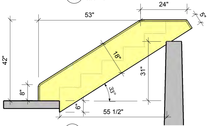
1 Right Side View A00 Scale: 1/2"=1'-0"
