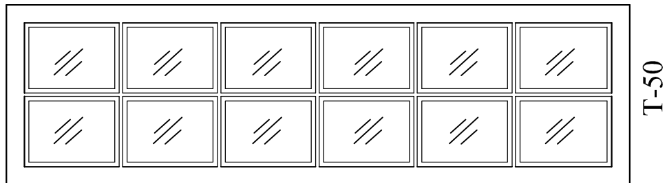
12 lite transom
