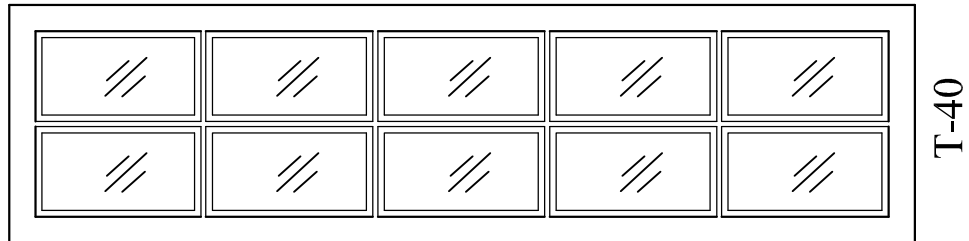
10 lite transom
