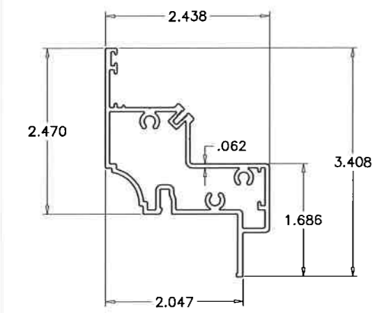
② VENT
