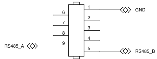
CONN DSUB 9-P MALE
