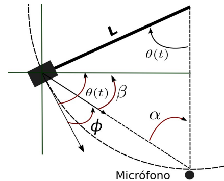
Figura 3. Esquema que permite identificar las relaciones entre los ángulos de la situación y a partir de ellas obtener el ángulo \varphi(t) en función de \theta(t) , este se puede generar con \omega_{\zeta}(t) y las condiciones iniciales.
