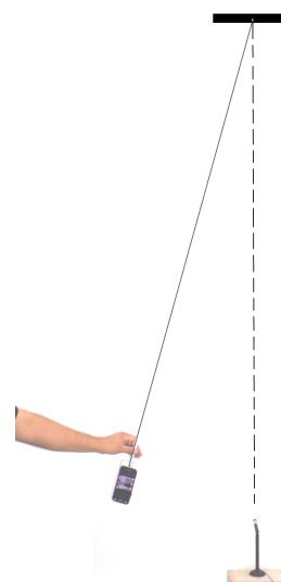
Figura 4. Esquema simplificado del dispositivo experimental. Se sujetan en el extremo inferior los teléfonos inteligentes y luego se deja oscilar el sistema.
