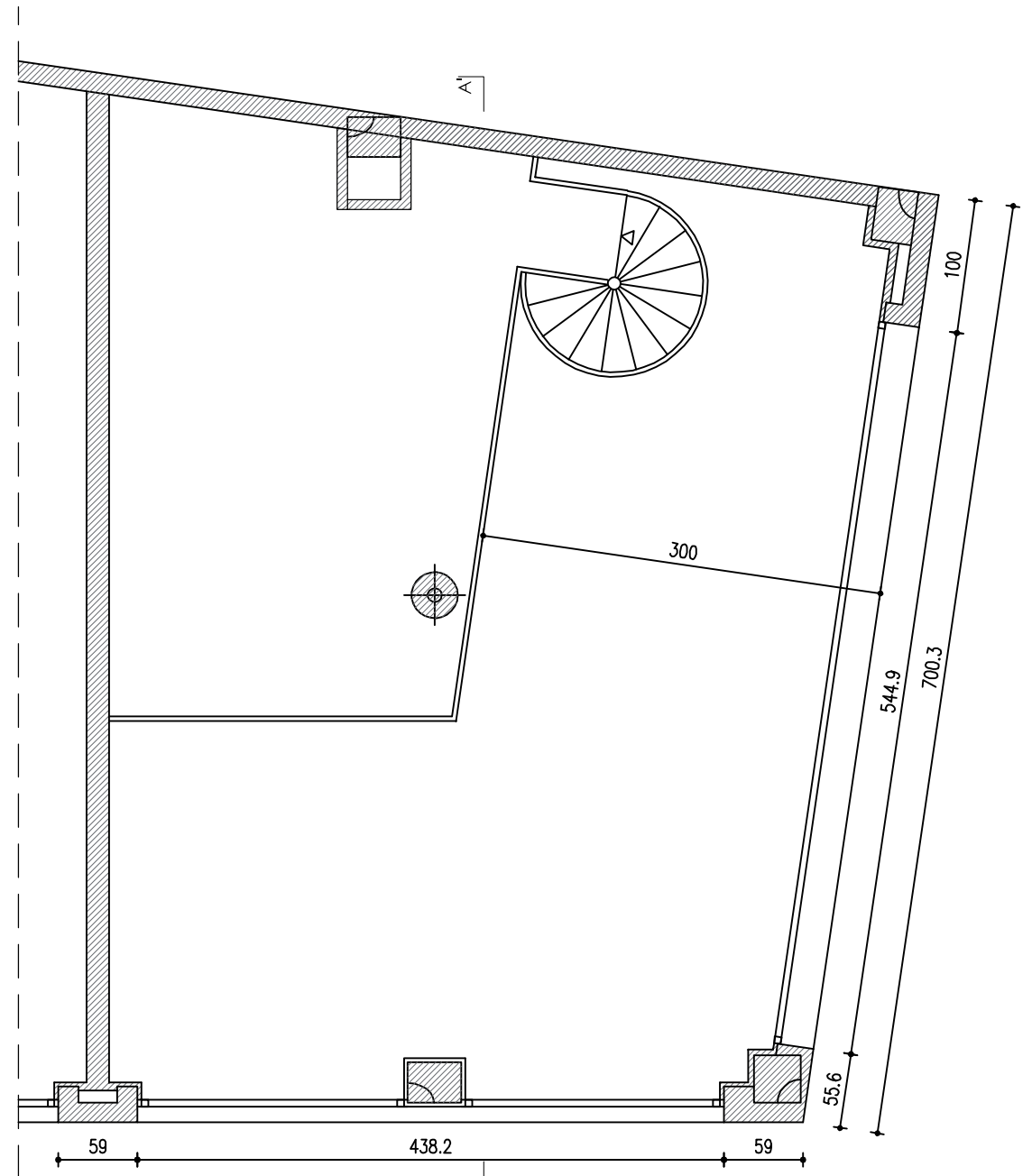
PLANTA ALTELL
