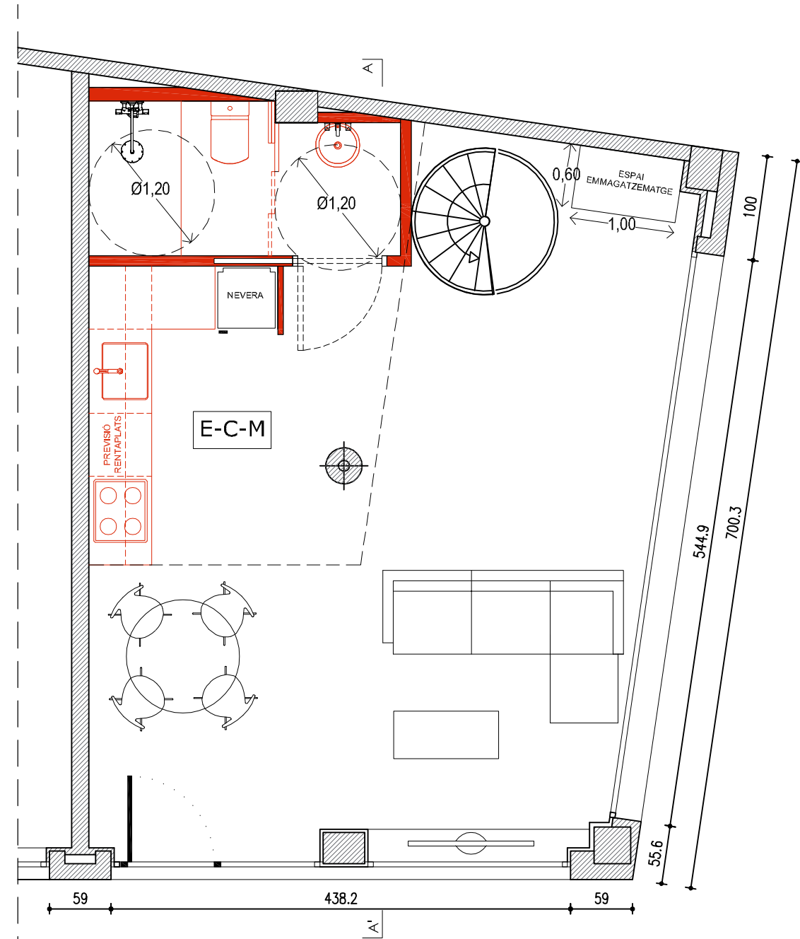
PLANTA BAIXA
