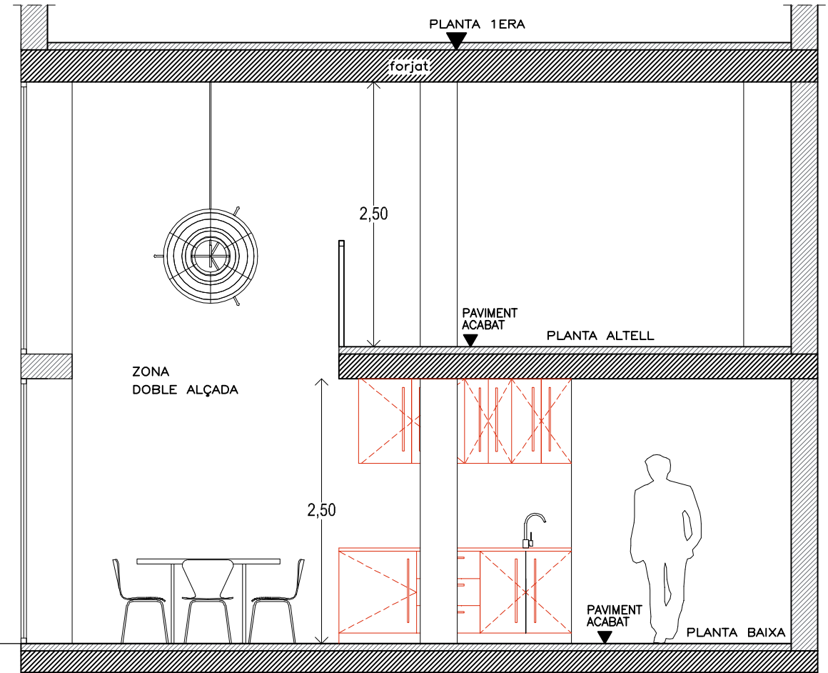
SECCIÓ A-A' PLANTA BAIXA
