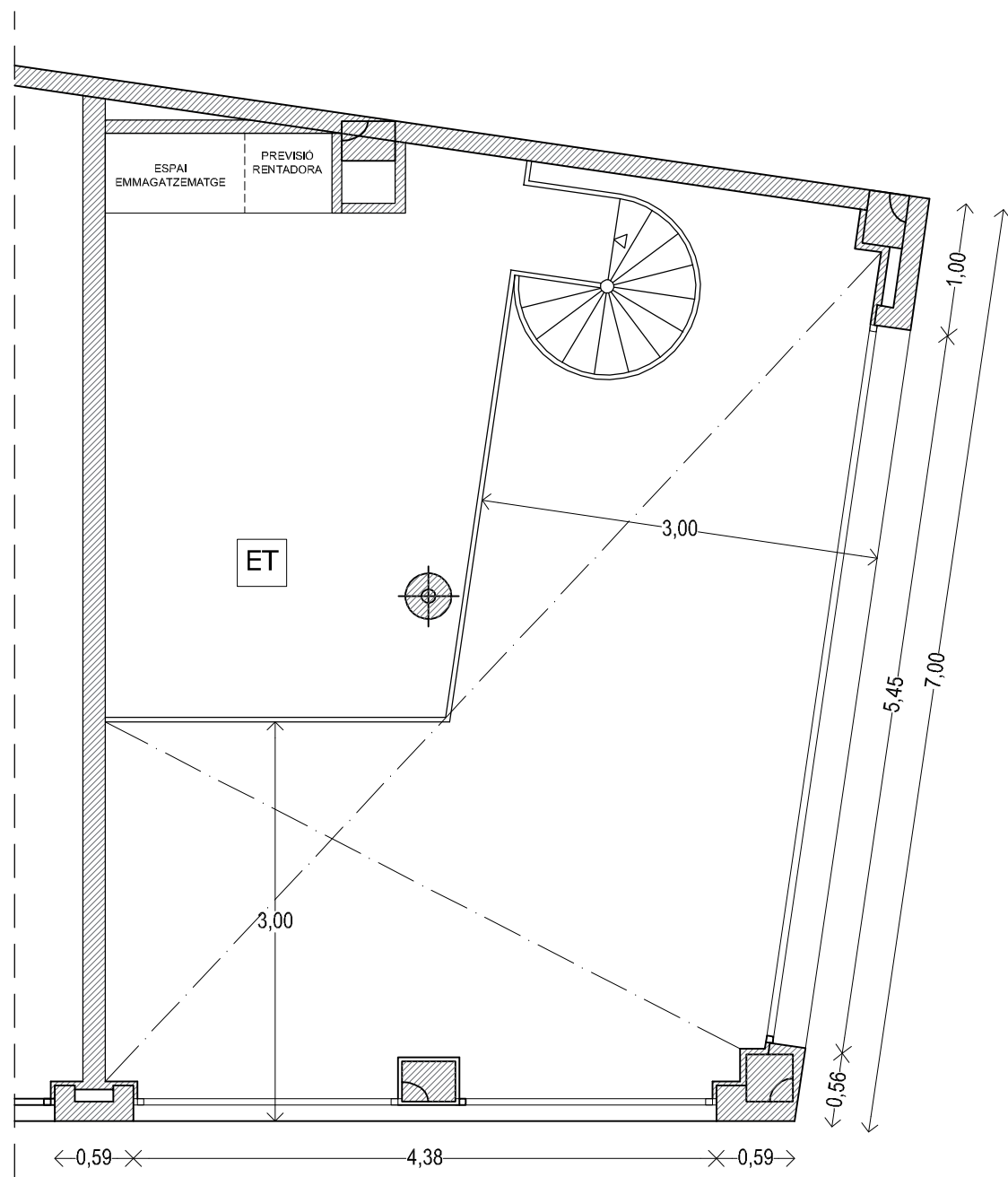
PLANTA BAIXA
