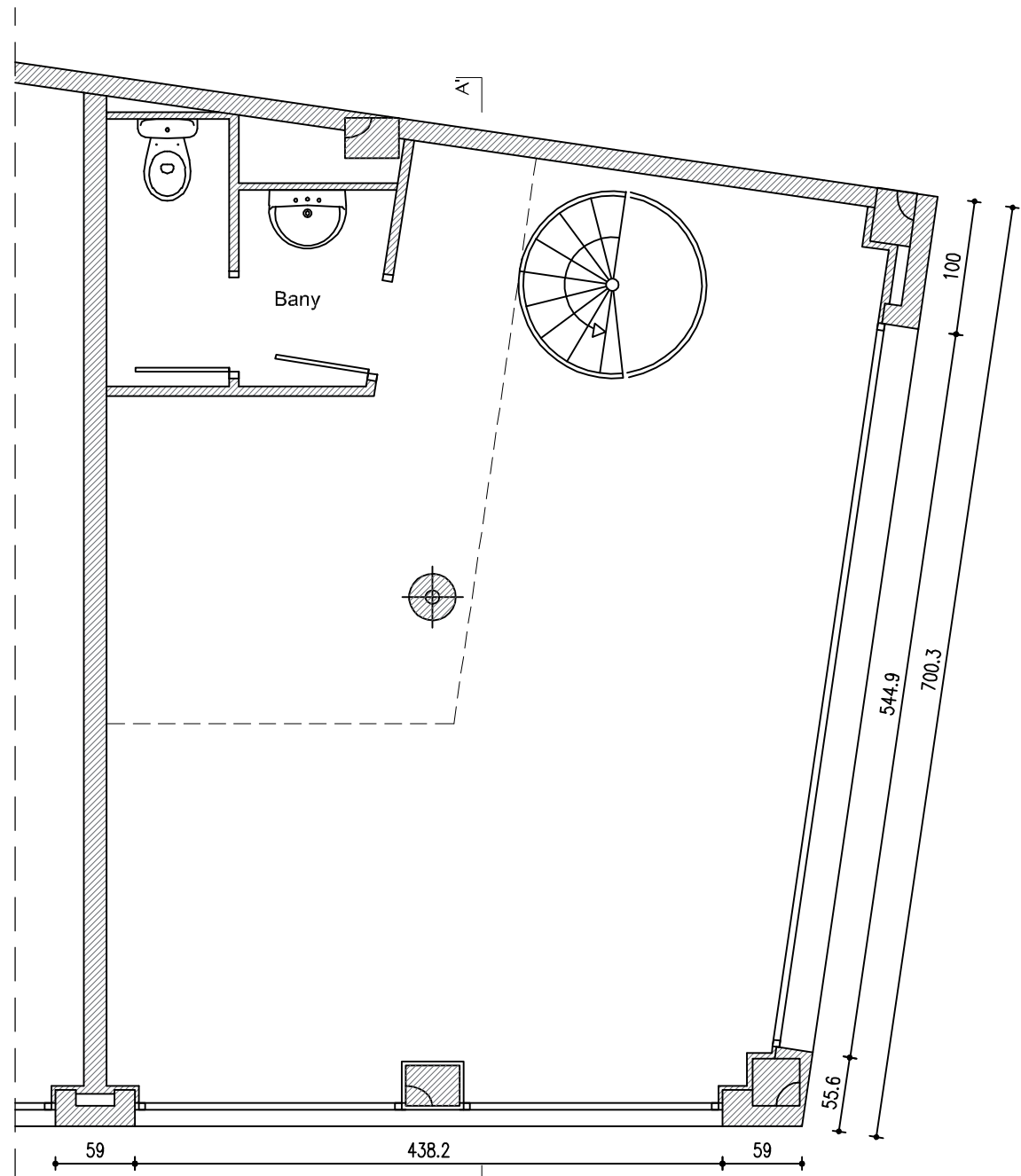
PLANTA BAIXA
