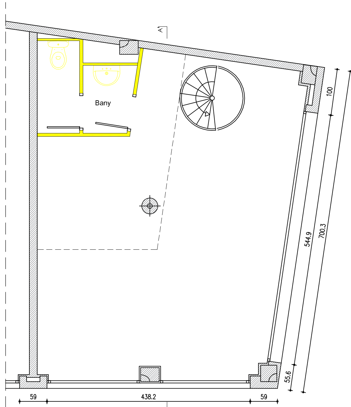
PLANTA BAIXA
