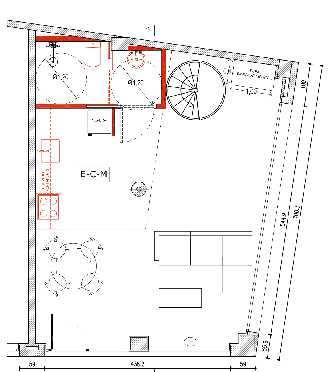
PLANTA BAIXA
