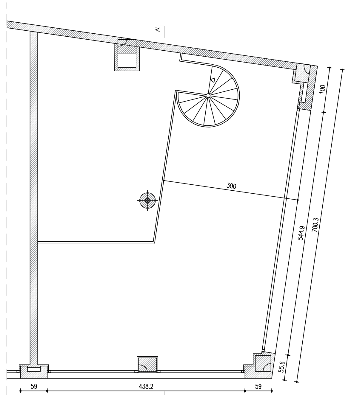
PLANTA ALTELL
