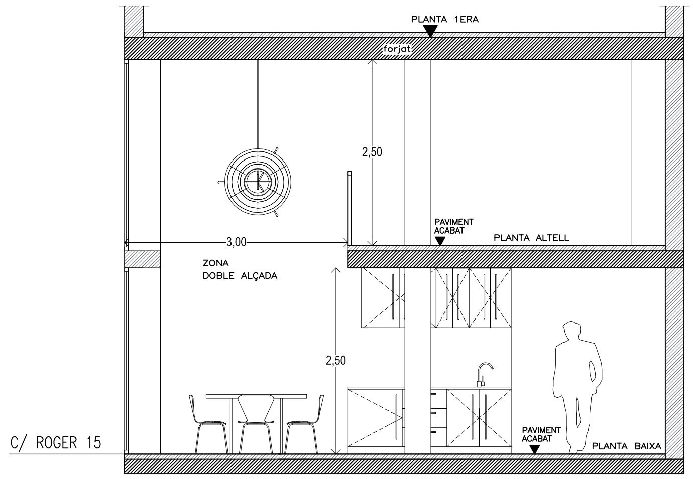
SECCIÓ A-A' PLANTA BAIXA
