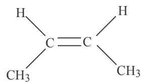
(Z)- بوت-2 إن
