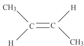
(E)- بوت-2 إن
