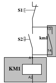
SCHEMA COMMANDE
